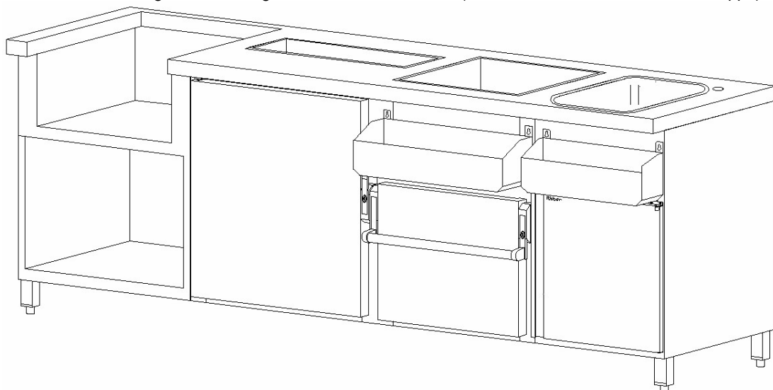
Abb.: Spül & Mix – Modul U Links mit 2 Speedracks
