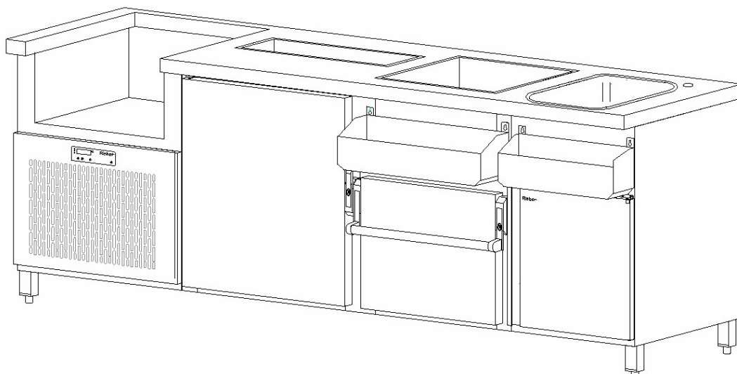
Abb.: Spül & Mix – Modul K Links mit 2 Speedracks
